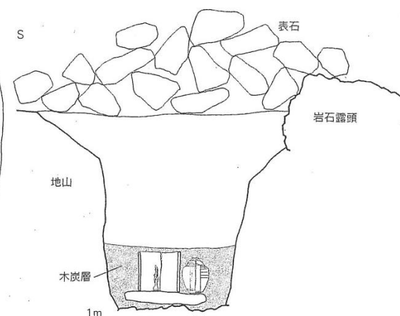
宝満A経塚埋置状況復原想定図 (1/4, 1/50)
