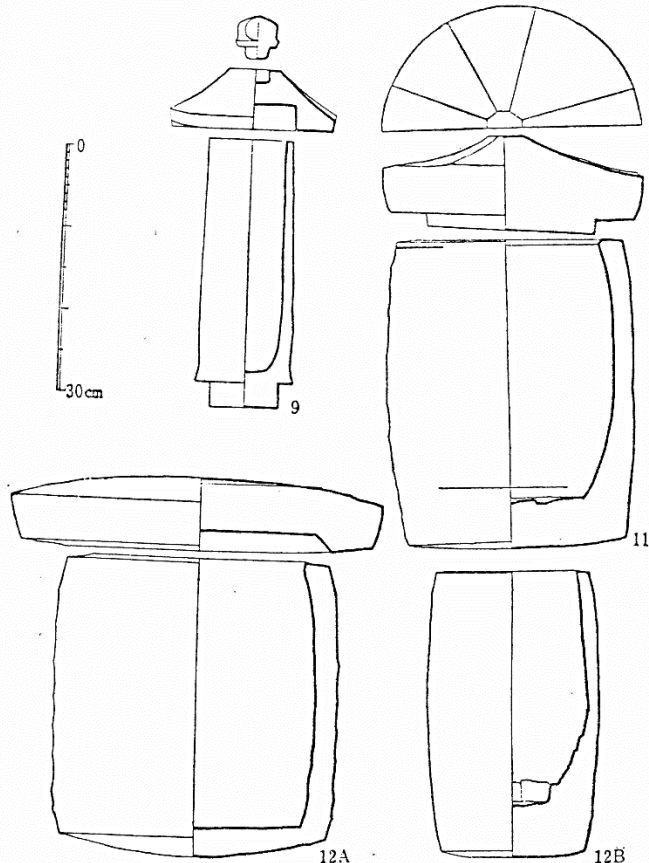
石製経筒実測図
